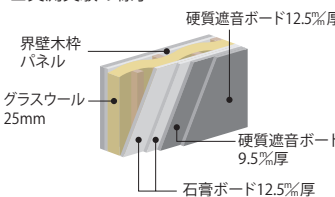
■界壁「ボイスカット仕様」イメージ図
