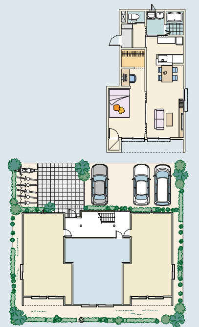
1LDK×6住戸 専有面積 45.13㎡ (13.65坪)
