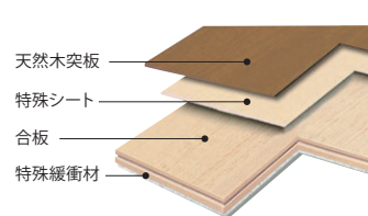
■遮音フローリング断面図
